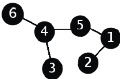
Figura 5 Degree (grados de centralidad), betweenness (intermediación) y 2-clanes
